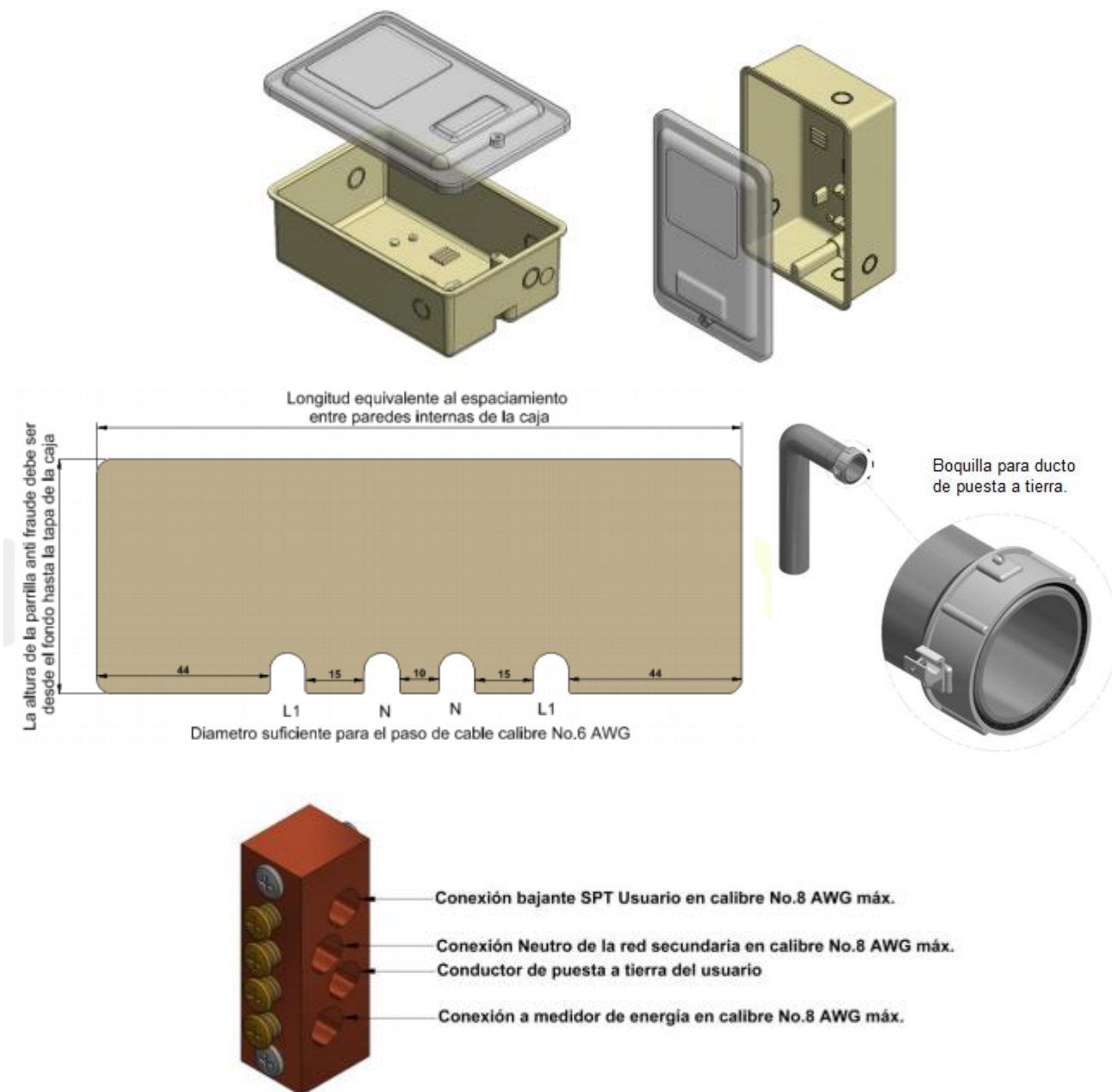
Figura 12. Caja polimérica para medidor de un puesto.
