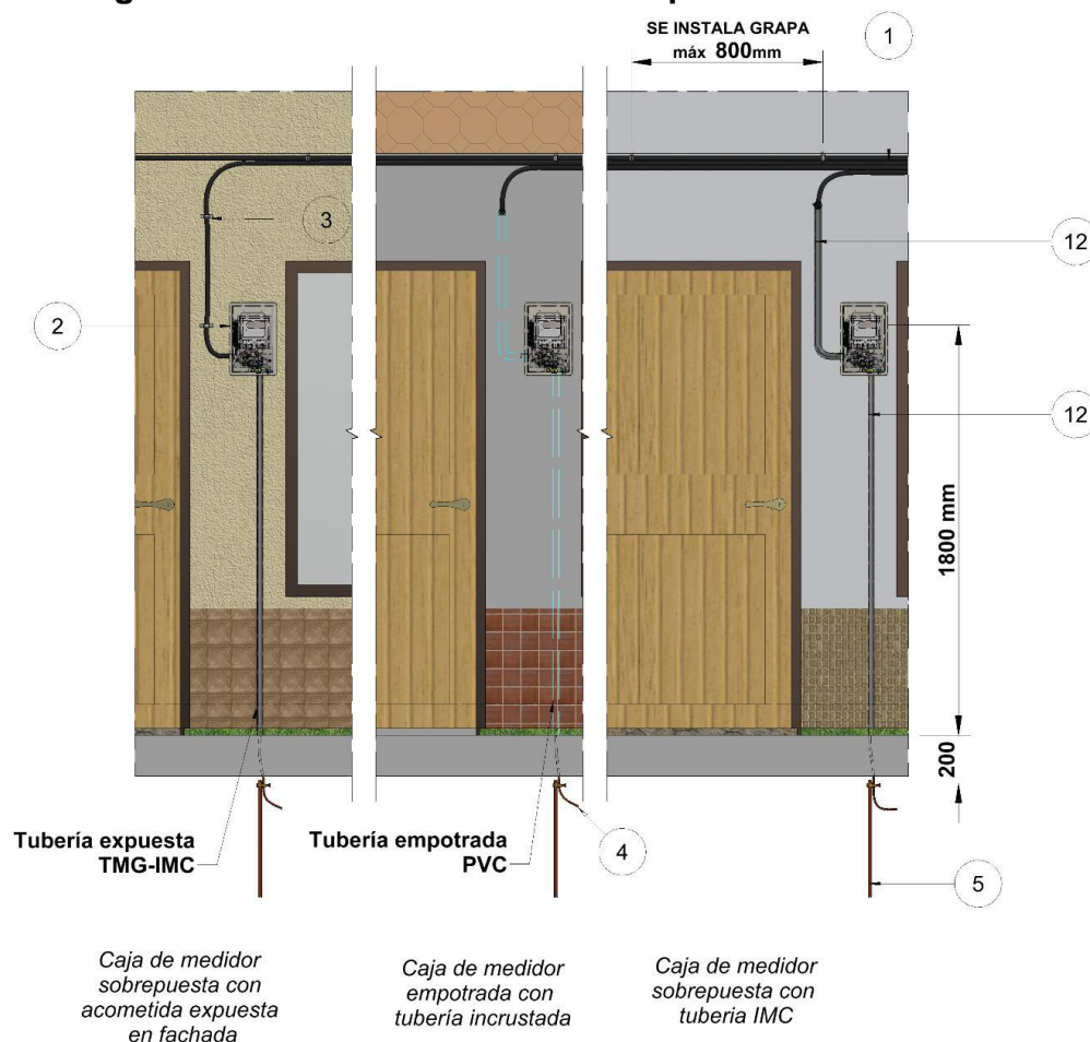
Figura 4. Acometida a la vista – Empotrada – En tubería.
