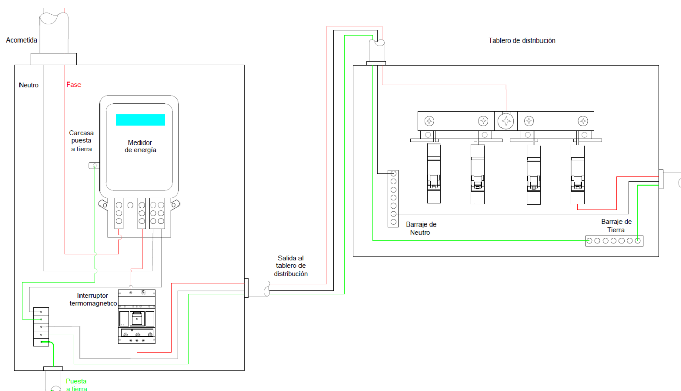
Figura 3. Conexión entre acometida y medidor
