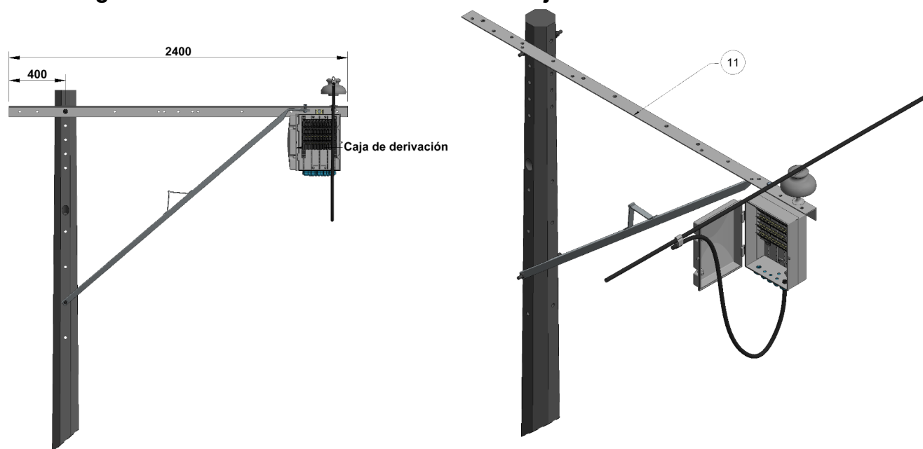
Figura 2. Derivación desde red aérea con caja de derivaciones en cruceta.
