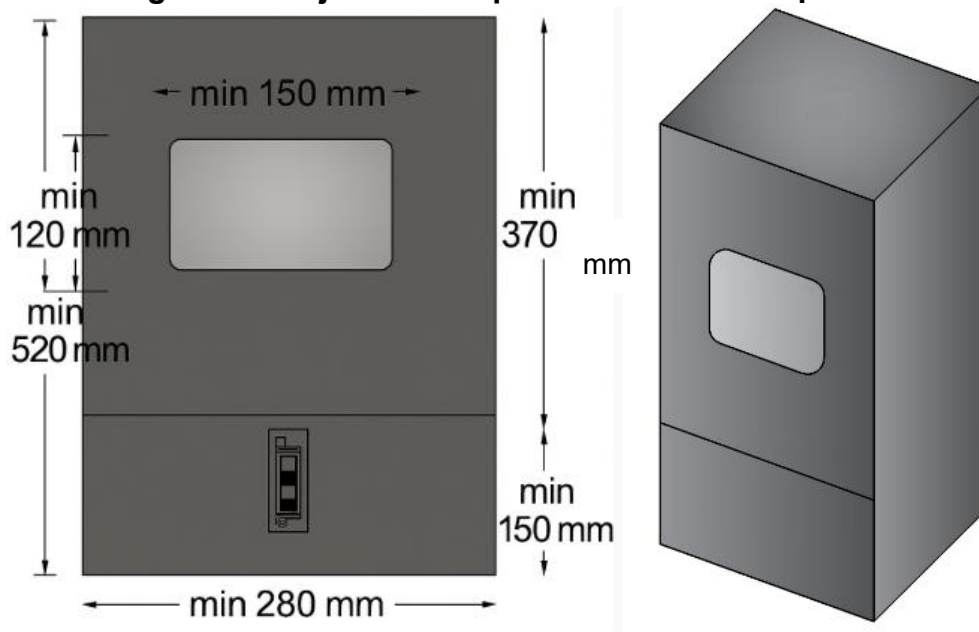
Figura 13. Caja metálica para medidor de un puesto.
